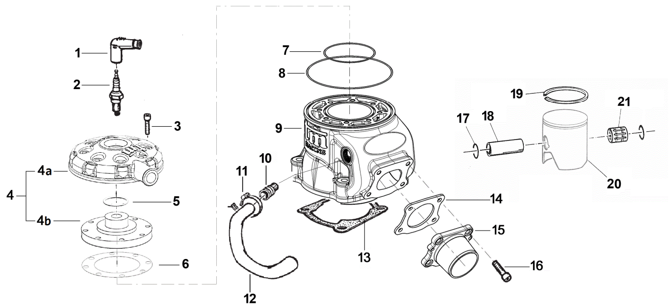
TAV. 01 – CILINDRO (Cylinder)
